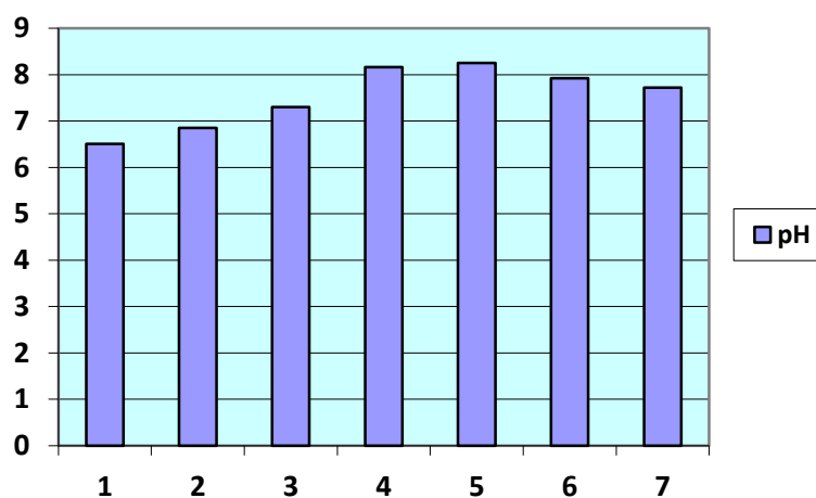
Диаграмма 3. Изменение pH талого снега от промышленной к жилой зоне
