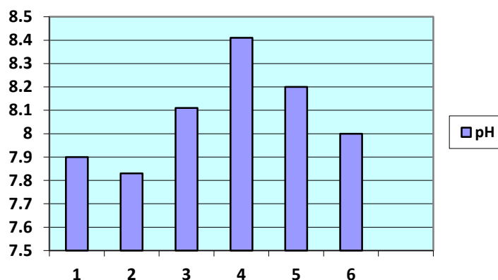
Диаграмма 4. Изменение рН талого снега на территории АЗС Красноармейского района
