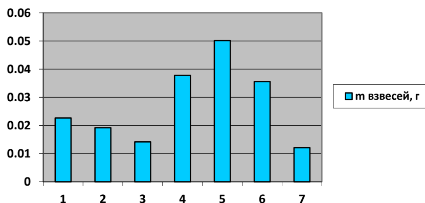
Диаграмма 1. Содержание твердых нерастворимых взвесей в пробах
