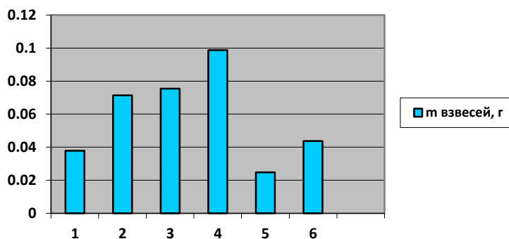
Диаграмма 2. Содержание твердых нерастворимых взвесей в пробах
