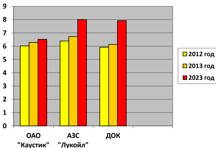
Диаграмма 5. Изменения количественных параметров значений рН талого снега в периоде с 2012 по 2023 год
